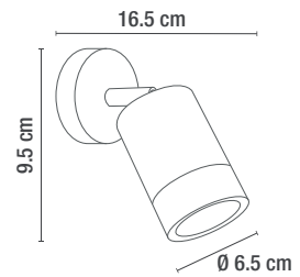
6316-GU10/GF
