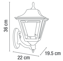
1501N
